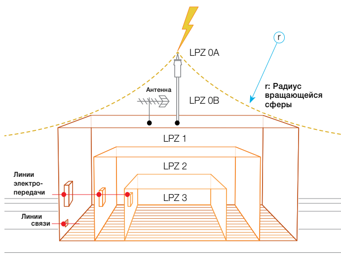
Внешняя система молниезащиты
