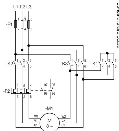
Схема включения
