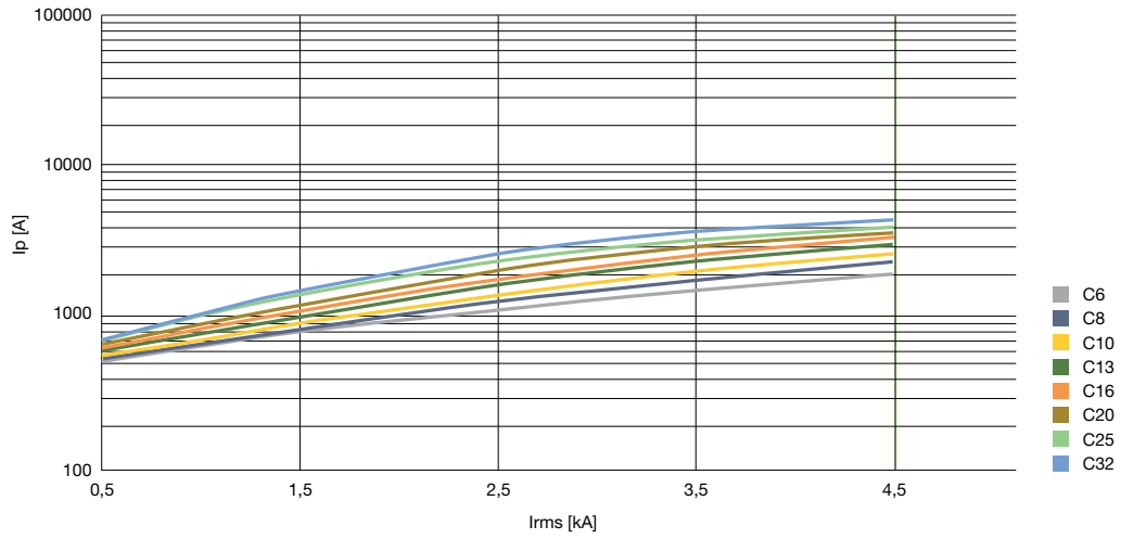
DS203NC L, характеристика C
