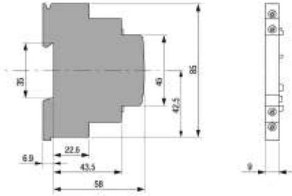
E293/X Модуль центрального ВКЛ/ВЫКЛ (одинаковое напряжение управления)
