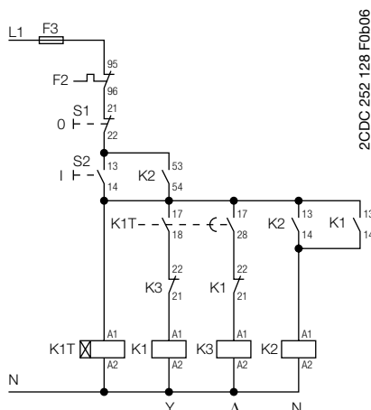
Схема управления
