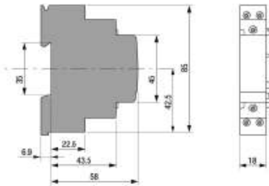
E294 Модуль центрального ВКЛ/ВЫКЛ (с различным напряжением управления)
