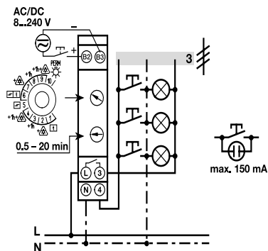
E 232E-8/230 Multi 10 3-проводная схема
