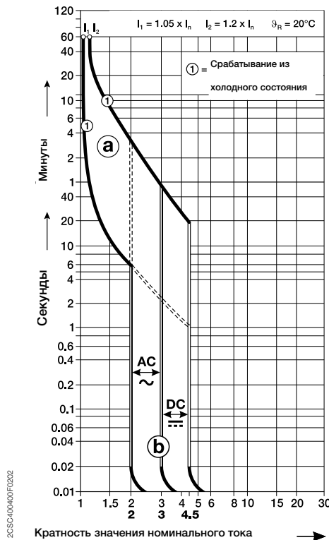
Характеристика Z IEC-EN60947-2
