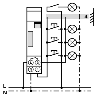
E 232-230 4-проводная схема
