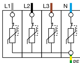
OVR T2 4L 40 275
