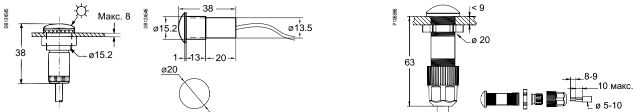
Фотоэлемент для щитового монтажа (15281) Крепится в вертикальном положении двумя винтами 2 Ø 4 мм снаружи щита
