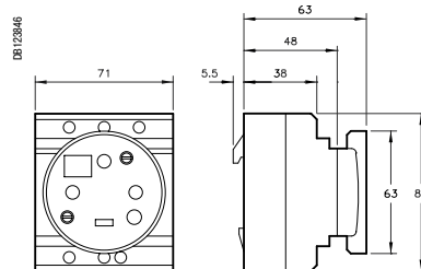
iPC 20 A
