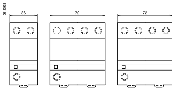
1P + N
