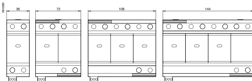
1P
