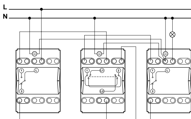
2 выключателя на два направления + 1 промежуточный выключатель с индикацией
