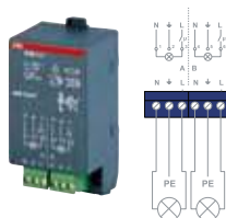
Модуль бинарного выхода, 2-канальный, 6 А, SA/M 2.6.1
