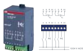
Модуль бинарного входа, 4-канальный, со сканированием контактов, BE/M 4.230.1
