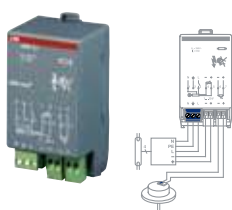
Модуль управления освещением, 1-канальный, 6 АХ, LRM 1.6.2
