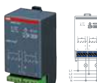
Модуль бинарного выхода, 2-канальный, 16 А, с сухими контактами, SA/M 2.16.1
