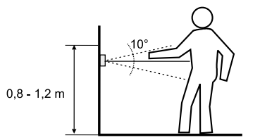
Зоны действия, горизонтальная и вертикальная (6815 U и 6816 U)
