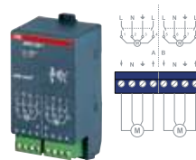
Модуль привода жалюзи, 2-канальный, 24 В, JA/M 2.24.1
