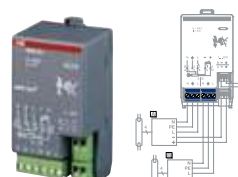
Активатор/светорегулятор, 2-канальный, 6 АХ SD/M 2.6.1
