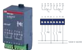
Модуль бинарного входа, 4-канальный, 12/24 В, BE/M 4.230.1
