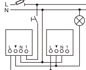
Параллельное подключение нескольких 6816 U
