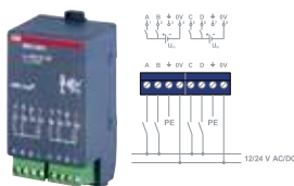
Модуль бинарного входа, 4-канальный, 230 В, BE/M 4.230.1
