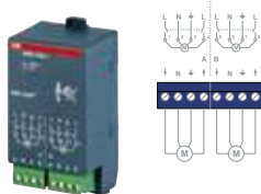
Модуль привода жалюзи, 2-канальный, 230 В, JA/M 2.230.1
