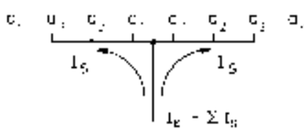
Поддача питания в центре шины
