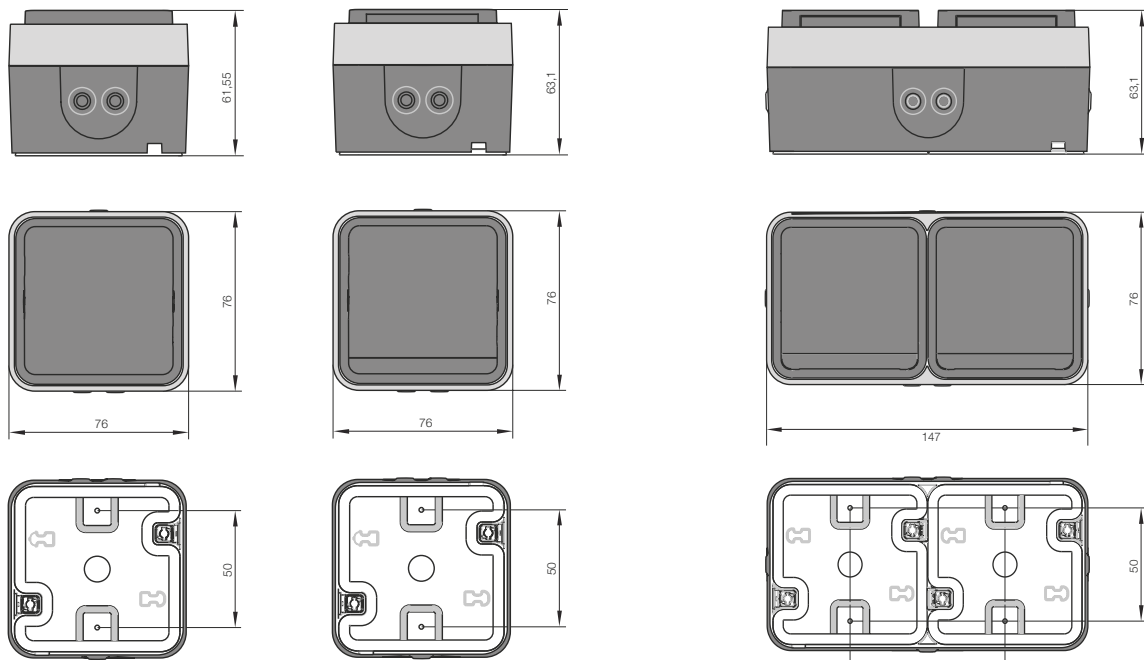
Рис 1: Выключатель/кнопка (слева), розетка SCHUKO с откидной крышкой (справа)
