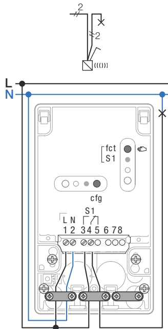
Рис 1: Переключение лампы
