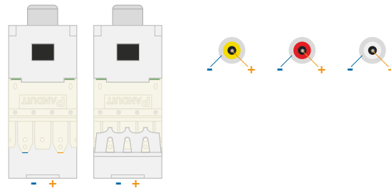
Рис 3: Разъем "тюльпан" Modul
