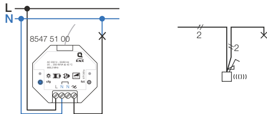
Рис 3: Светорегулировка лампы
