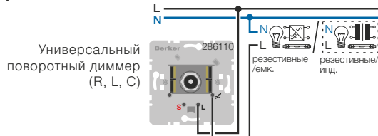
Рис 1: Выключение
