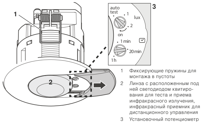
Рис 1: Обзор устройств
