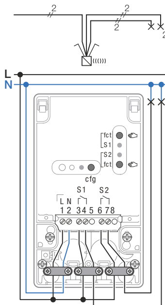
Рис 2: Переключение 2 ламп
