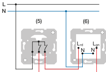
Рис 3: Пример подключения светодиодной сигнальной подсветки, красное/зеленое освещение
