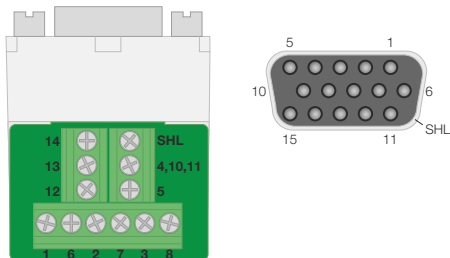
Рис 1: Модуль VGA
