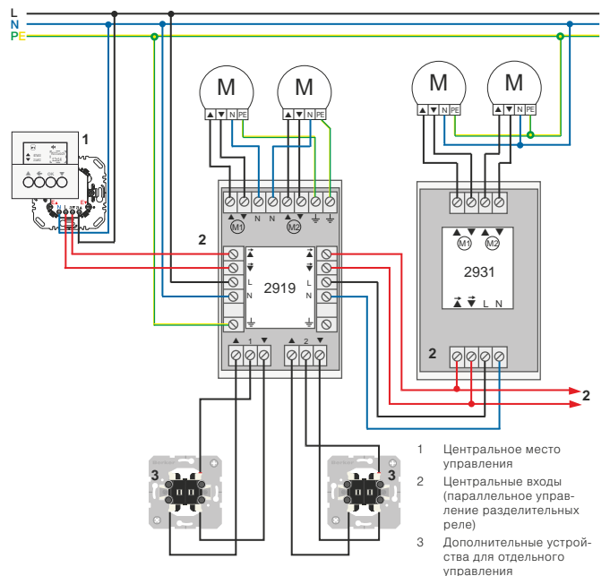
Рис 3: Схема подсоединения разделительного реле REG
