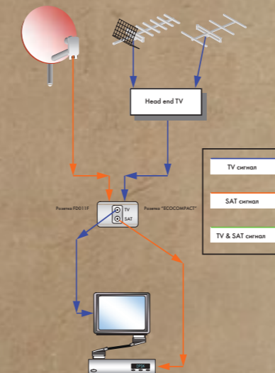
ПРИМЕР ИСПОЛЬЗОВАНИЯ РОЗЕТКИ FD011F ИЛИ КОМПЛЕКТА „ЕКОСОМРАСТ“ ДЛЯ СОЗДАНИЯ СЕТИ ТВ/СПУТНИК
