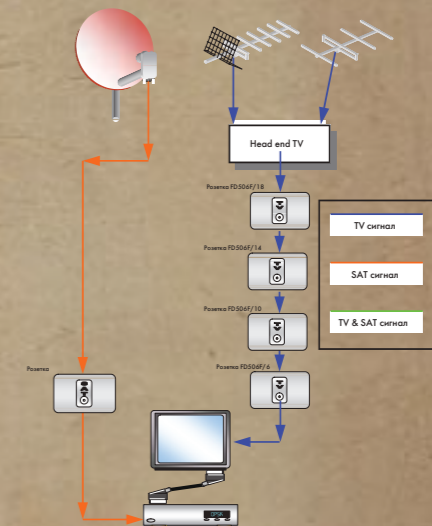
ПРИМЕР ИСПОЛЬЗОВАНИЯ РОЗЕТОК FD506F И FD002F ДЛЯ СОЗДАНИЯ „ПРОХОДНОЙ“ ТВ-СЕТИ И НЕПОСРЕДСТВЕННОГО ПОДКЛЮЧЕНИЯ СПУТНИКОВОГО ТВ
