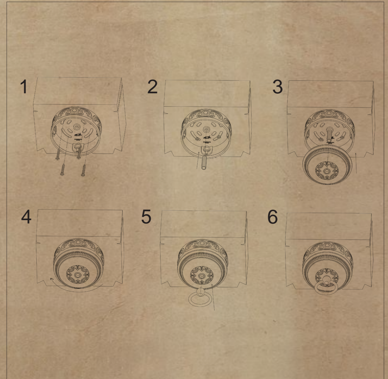
Схема монтажа подвеса люстр для наружного монтажа.
