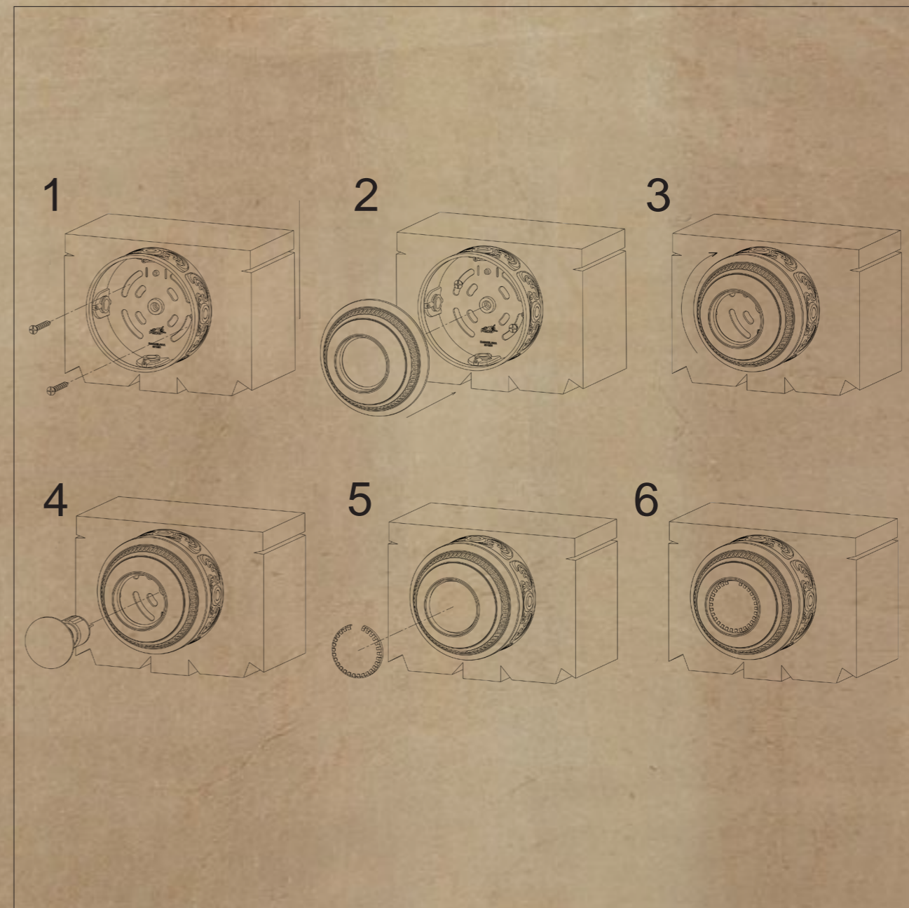
Схема монтажа наружного светильника. В светильник могут устанавливаться, как лампы накаливания, так и светодиодные лампы.
