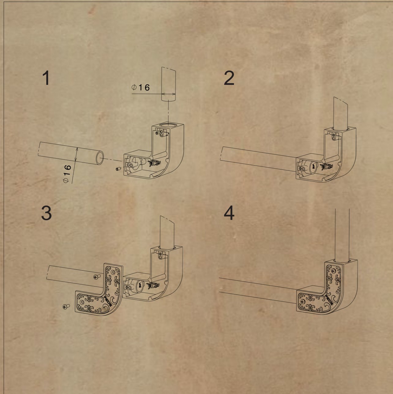
Схема подсоединения труб диаметром 16мм. к универсальному аксессуару «Угол 90 градусов»
