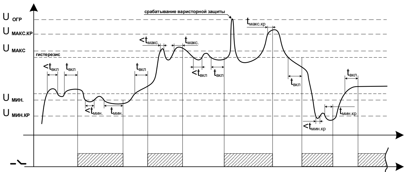
Рис. 1а. Защита по напряжению (по любой фазе)
