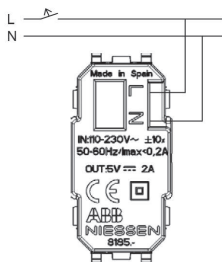
Рис. 1. Схема 8185.2
