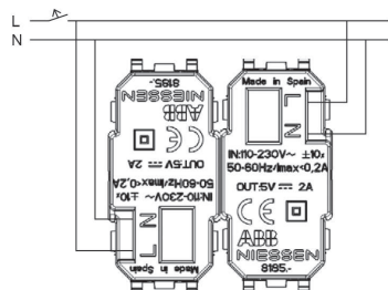
Рис. 2. Схема 8185.3
