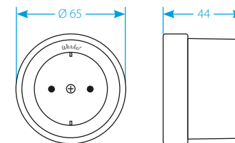
Розетки металлические
