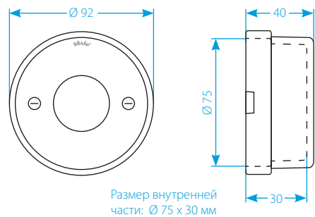
Распределительная коробка
