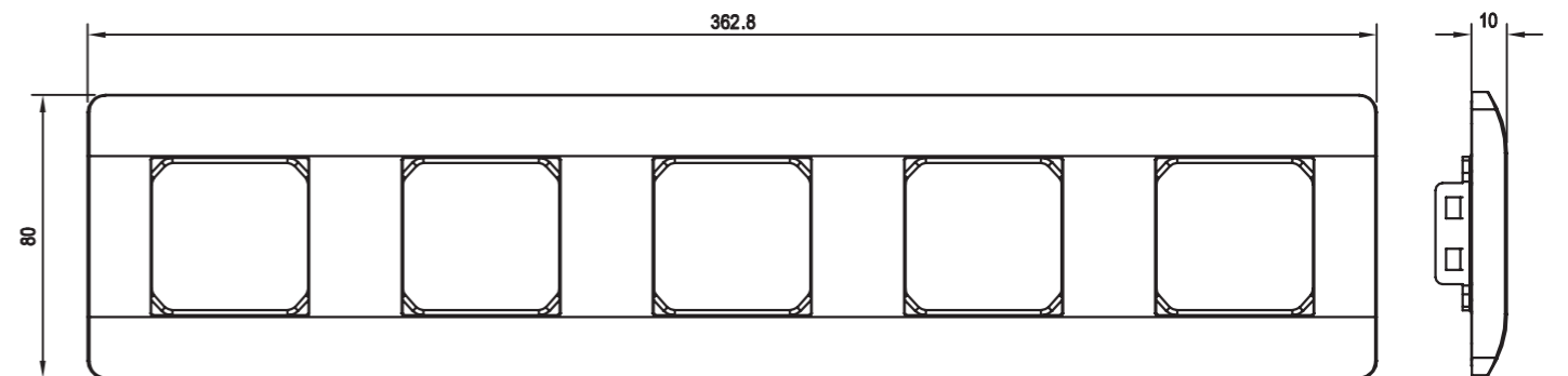
Рамка 5-постовая
