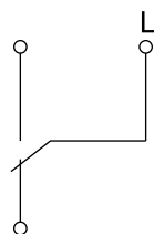
Выключатель одноклавишный проходной
