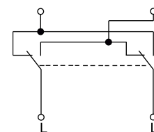
Переключатель одноклавишный
