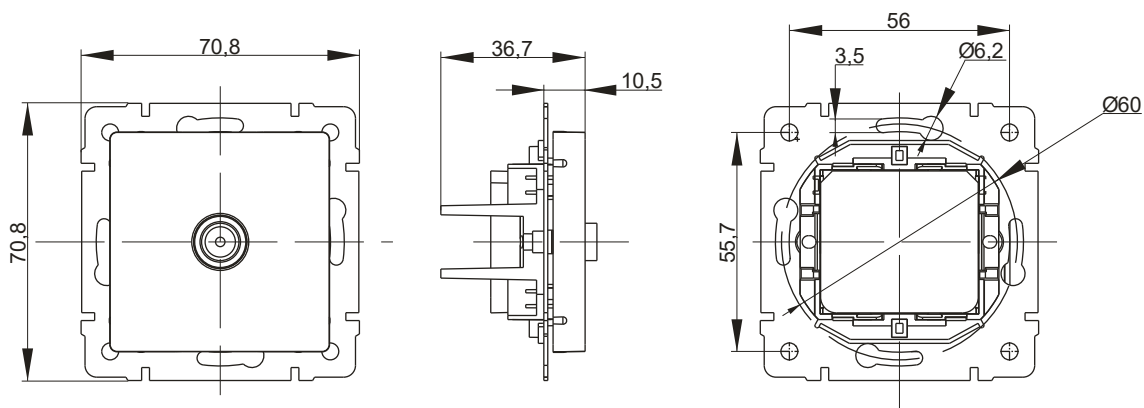
Телевизионная розетка
