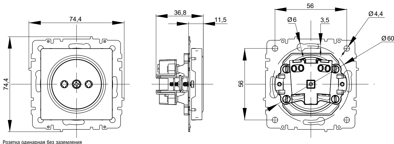
Розетка одинарная без заземления
