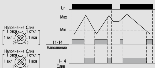
Диаграмма работы реле ORL-02 в режиме контроля двух уровней
