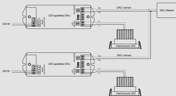
Схема установки 5
