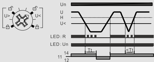
Реле ORV-01. Режим пониженного напряжения без блокировки
