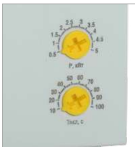
На лицевой панели – регуляторы ограничения мощности и времени включения нагрузки.
