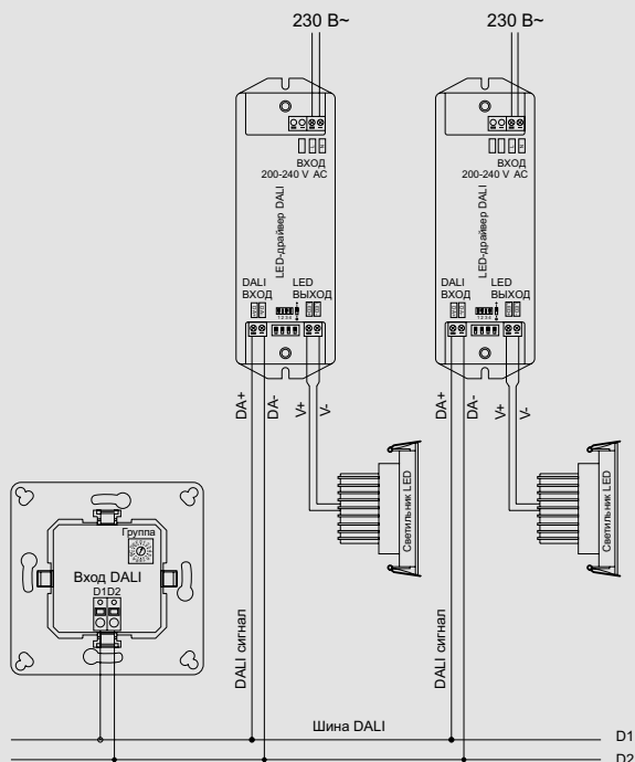
Схема установки 4
